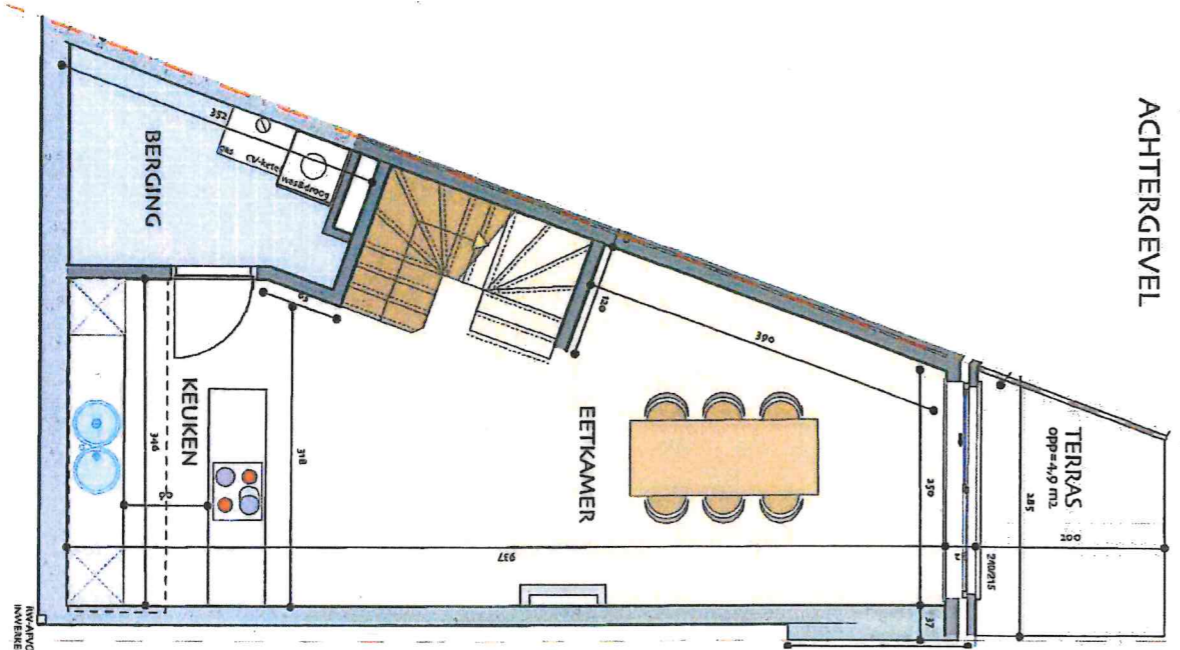
NIVEAU -1
